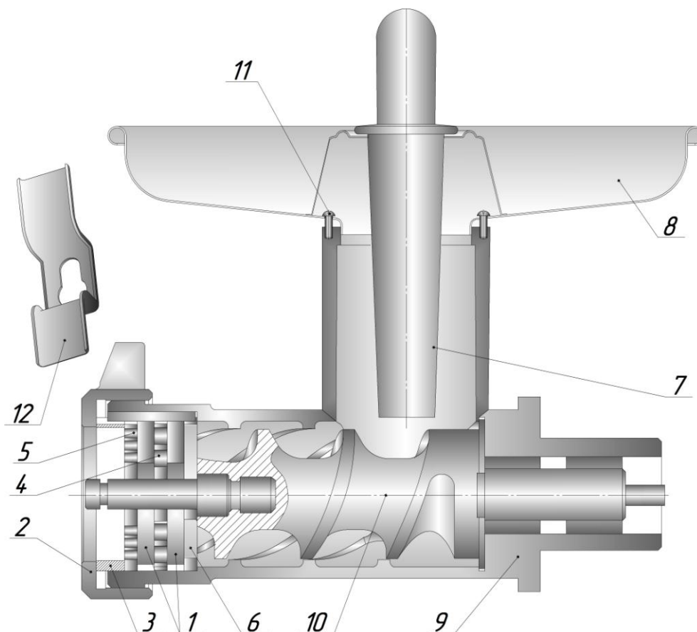
Рисунок 2 – Мясорубка ММ
