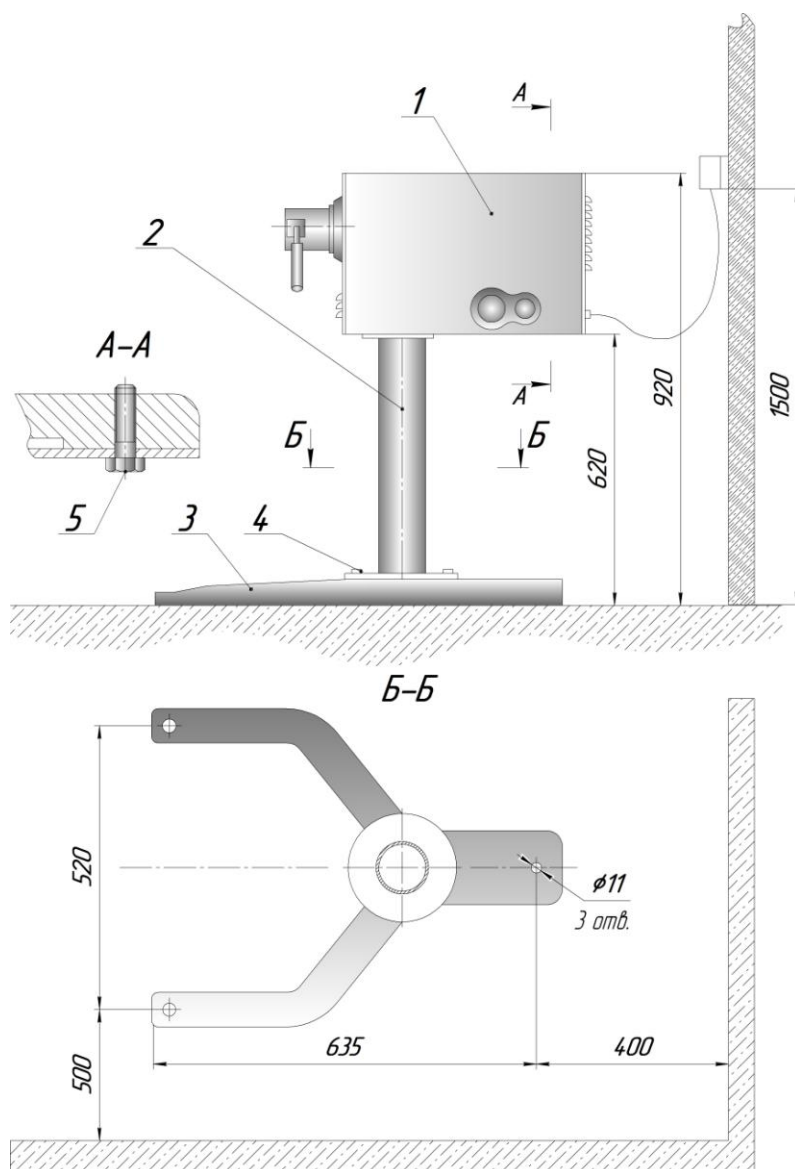
Рисунок 11 – Установка приводного механизма ПМ на подставке П-01 1– приводной механизм, 2 – стойка, 3 – опора, 4 и 5 – болты.
