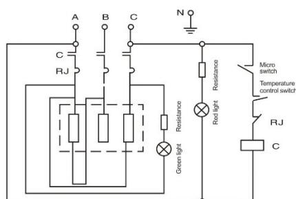
3 фазы 380В
