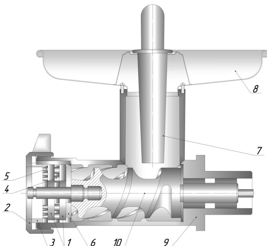
Рисунок 4 – Насадка мясорубки
