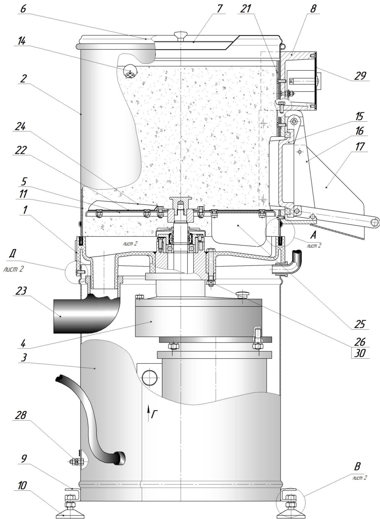
Рисунок – 1 Машина картофелеочистительная К-200 (лист 1)
